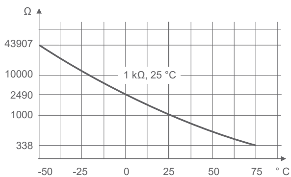
fig. 2 - Valeur ohmique des sondes
