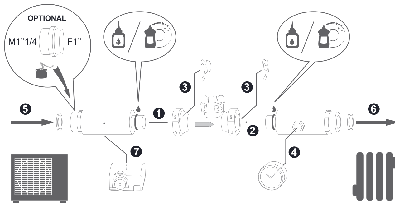
fig. 6 - Montage des tuyauteries et débitmètre
