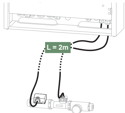
fig. 16 - Raccordement débitmètre et sonde départ chauffage
