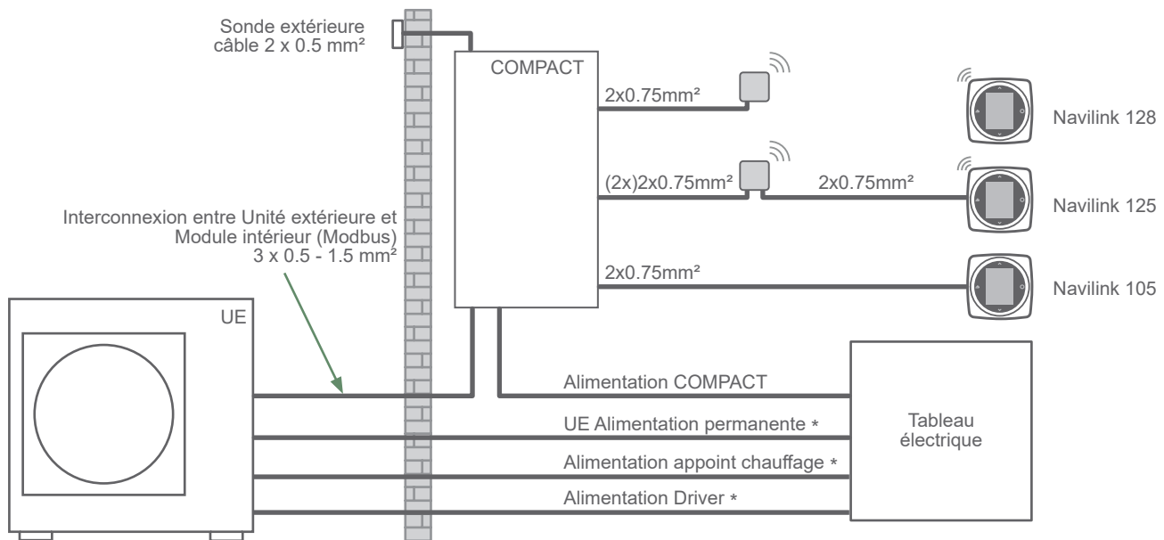
fig. 7 - Schéma d'ensemble des raccordements électriques pour une installation simple
