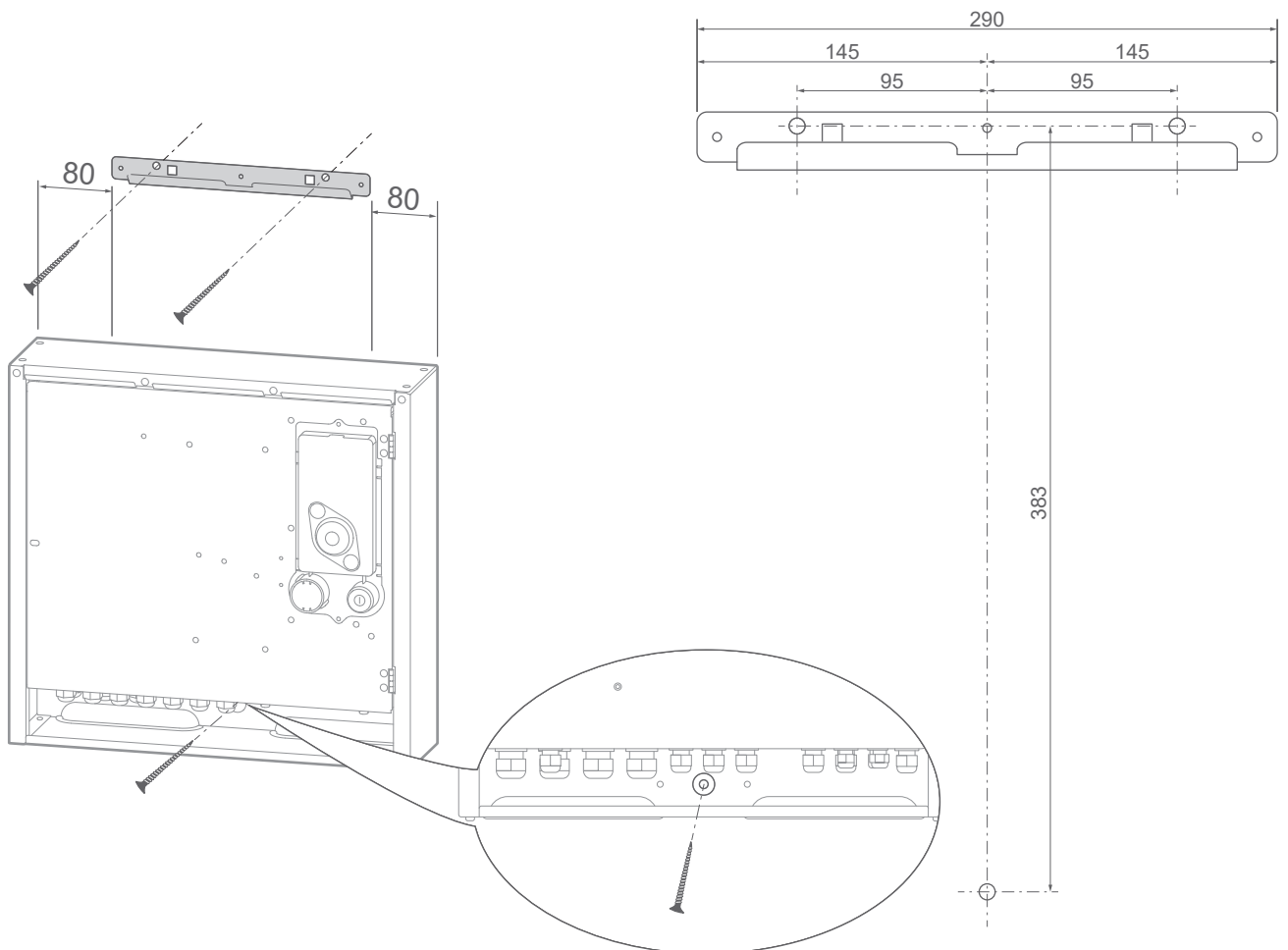
fig. 4 - Fixation du support
