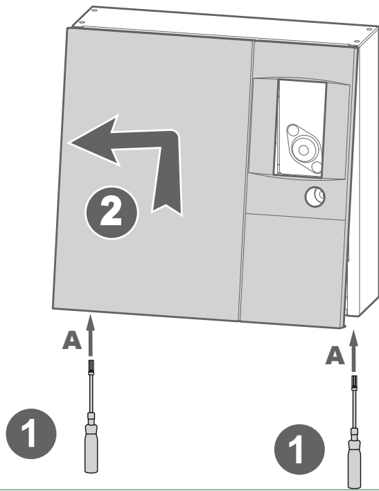
fig. 5 - Dépose de l'habillage
