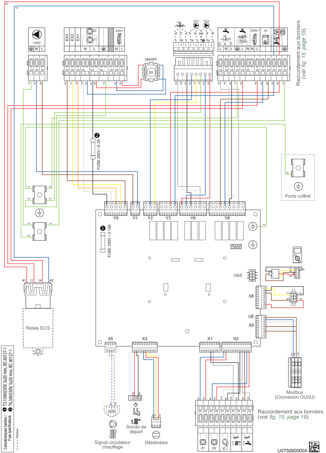
fig. 22 - Câblage électrique Module intérieur (hors raccordements installateur)
