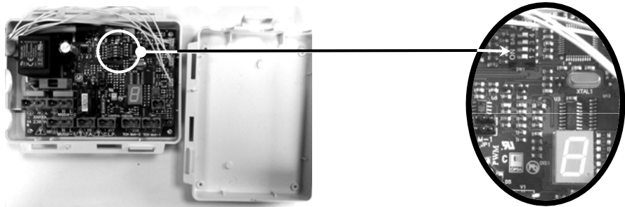
Ouvrir le module et régler le canal avec les switches
